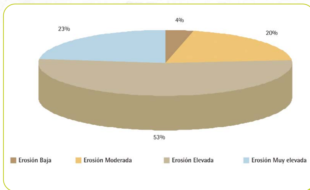
SUELO SEGÚN EROSIÓN. GUADALTEBA
